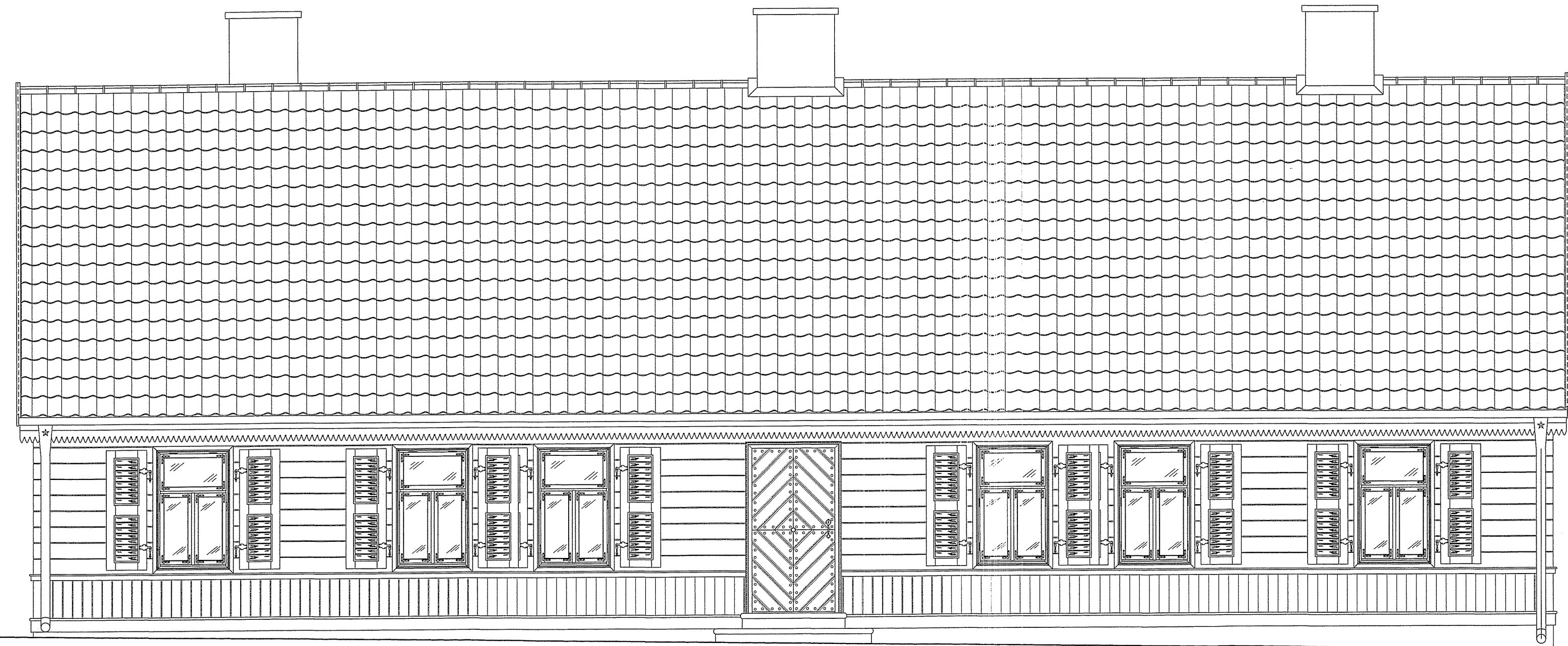
ELEWACJA PÓŁNOCNO - WSCHODNIA
